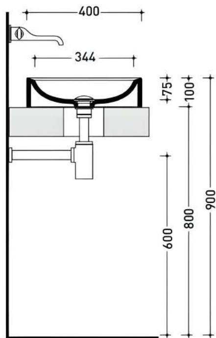
sezione longitudinale / section
