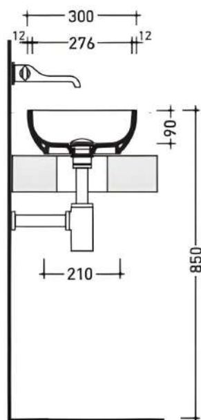
sezione longitudinale / section
