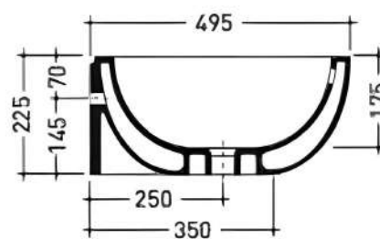
sezione longitudinale / section
