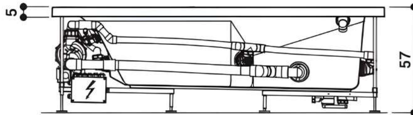
Left hand version view · Abb. Linksausführung
